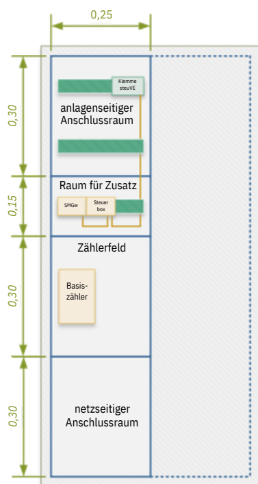
Abbildung 3 – Zählerschrank eHz (BKE)
