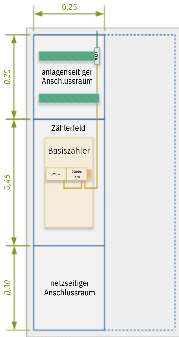
Abbildung 2 – Zählerschrank 3.Hz (DPA)
