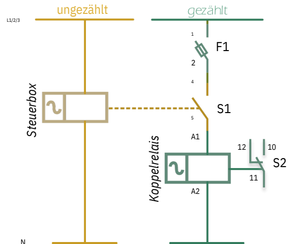
Abbildung 7 – Schematische Darstellung der Ansteuerung
