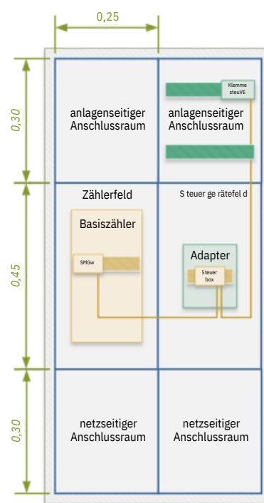
Abbildung 5 – Zählerschrank 3.Hz inkl. Steuergerätefeld (nur bei Bestand)
