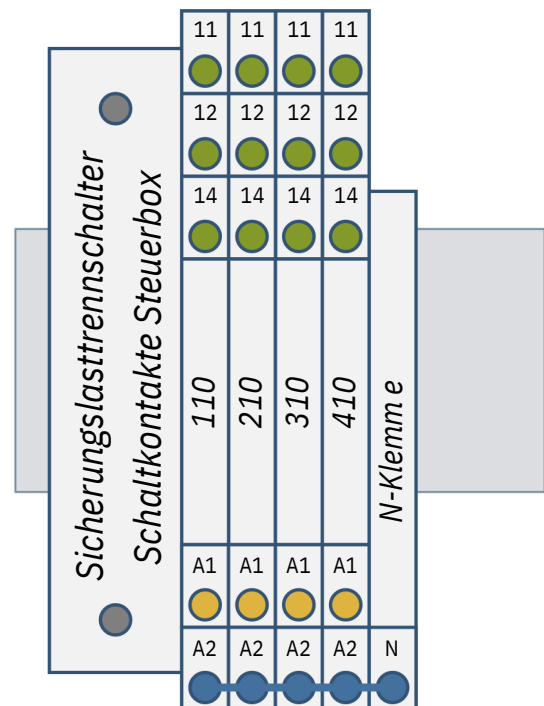
Abbildung 6 - Beispiel Aufbau der Koppelrelais
