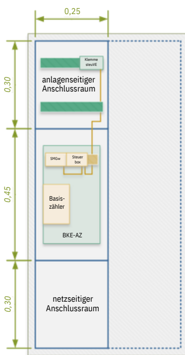
Abbildung 4 – Zählerschrank 3.Hz
