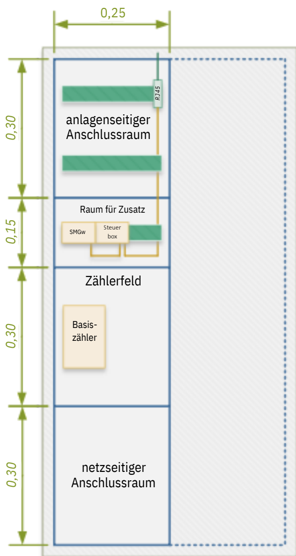
Abbildung 1 – Zählerschrank eHz (BKE)
